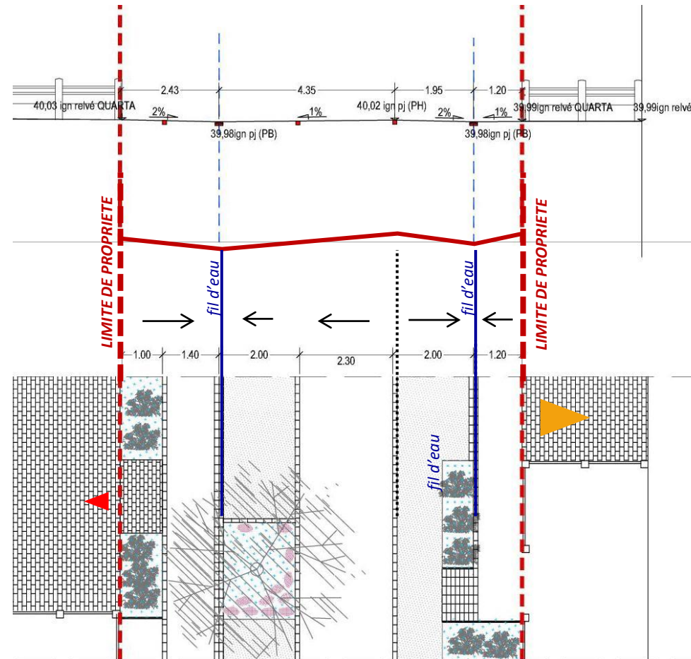
Profil chaussé projet
